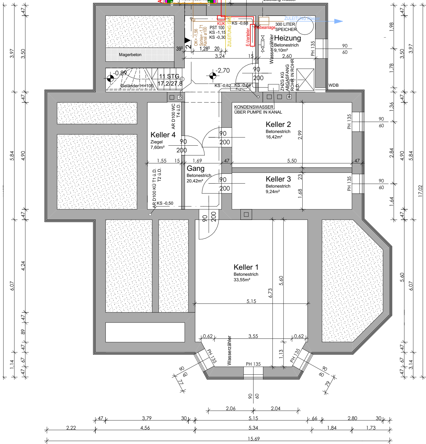
KELLERGESCHOSS M 1:100
