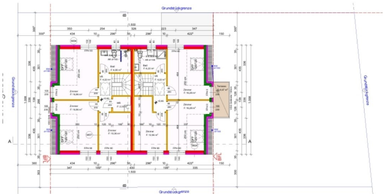
1.DACHGESCHOSS
