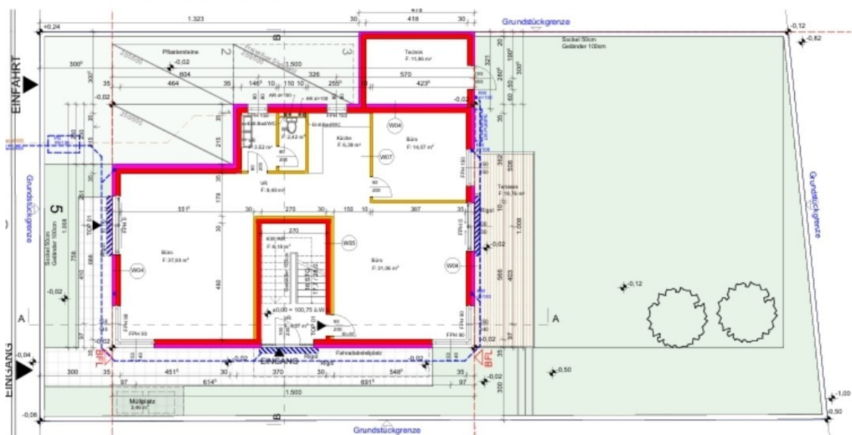
ERDGESCHOSS
