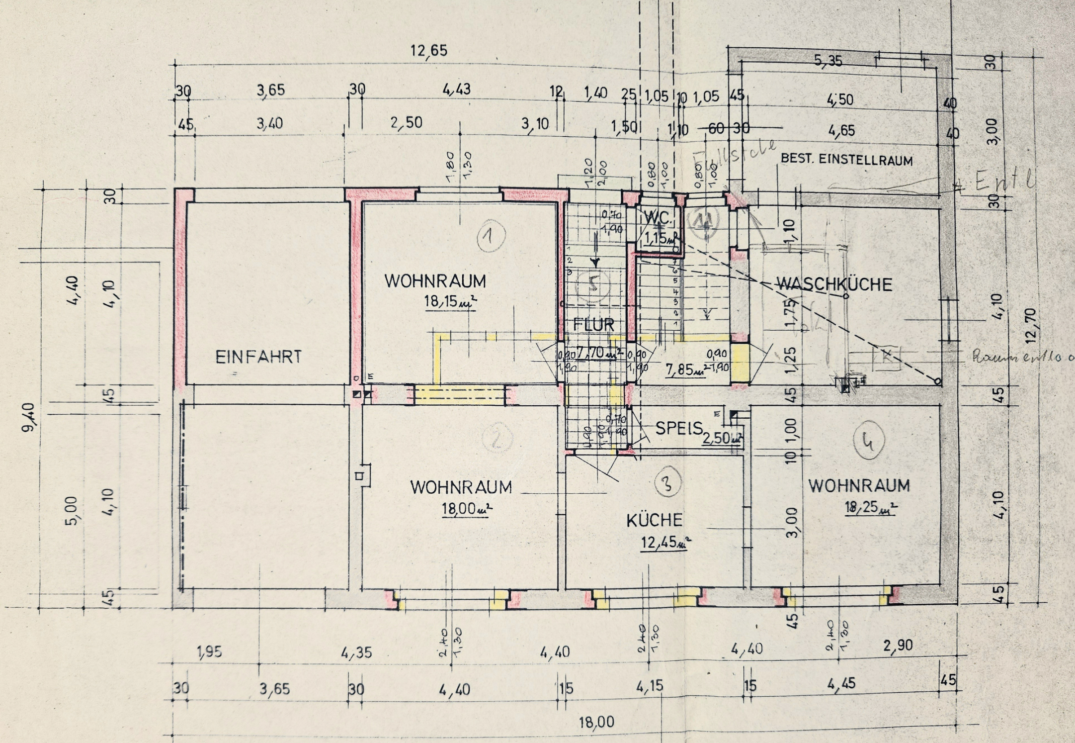
ERDGESCHOSSGRUNDRISS
