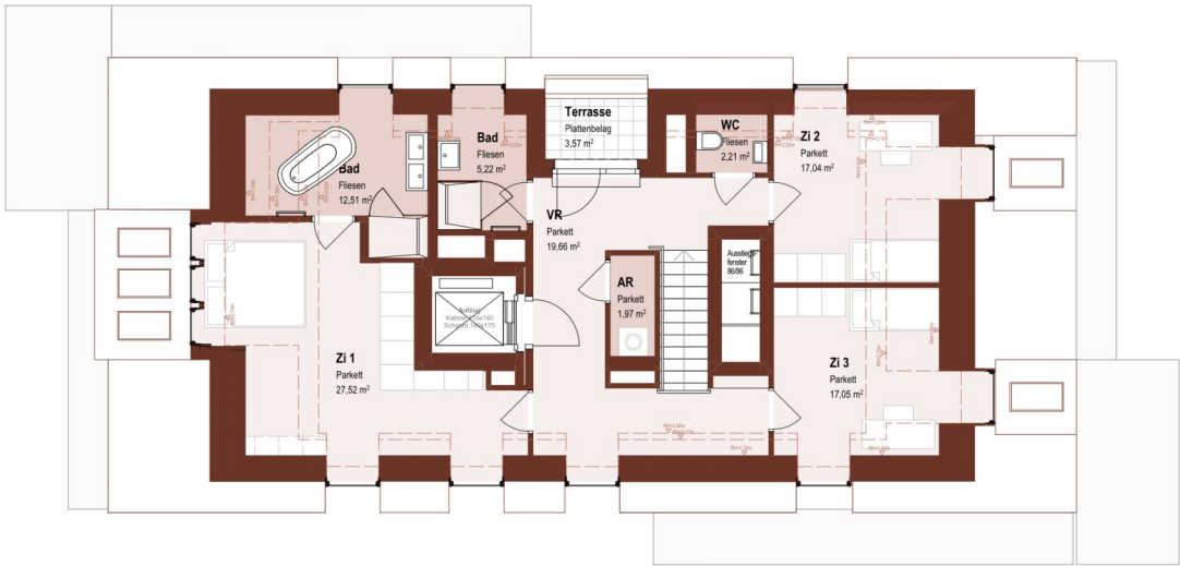
2.Dachgeschoss
