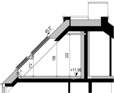
Schnitt 20.A
