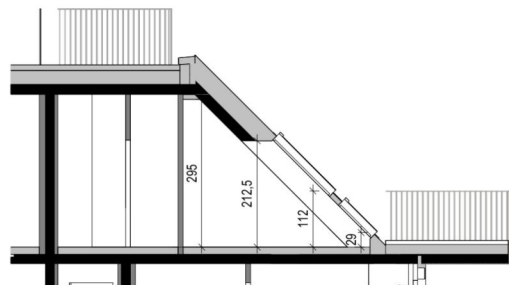
Schnitt 33.A
