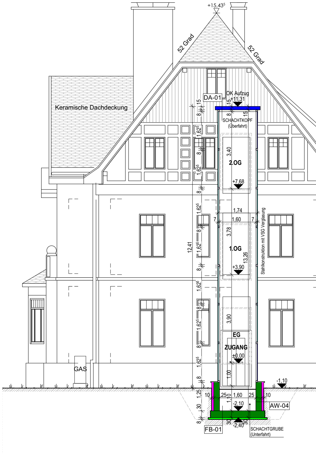
SCHNITT 1-1 M 1:100
