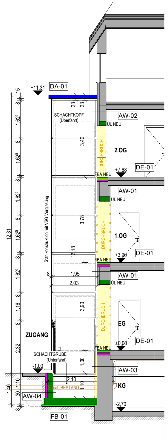
SCHNITT 2-2 M 1:100
