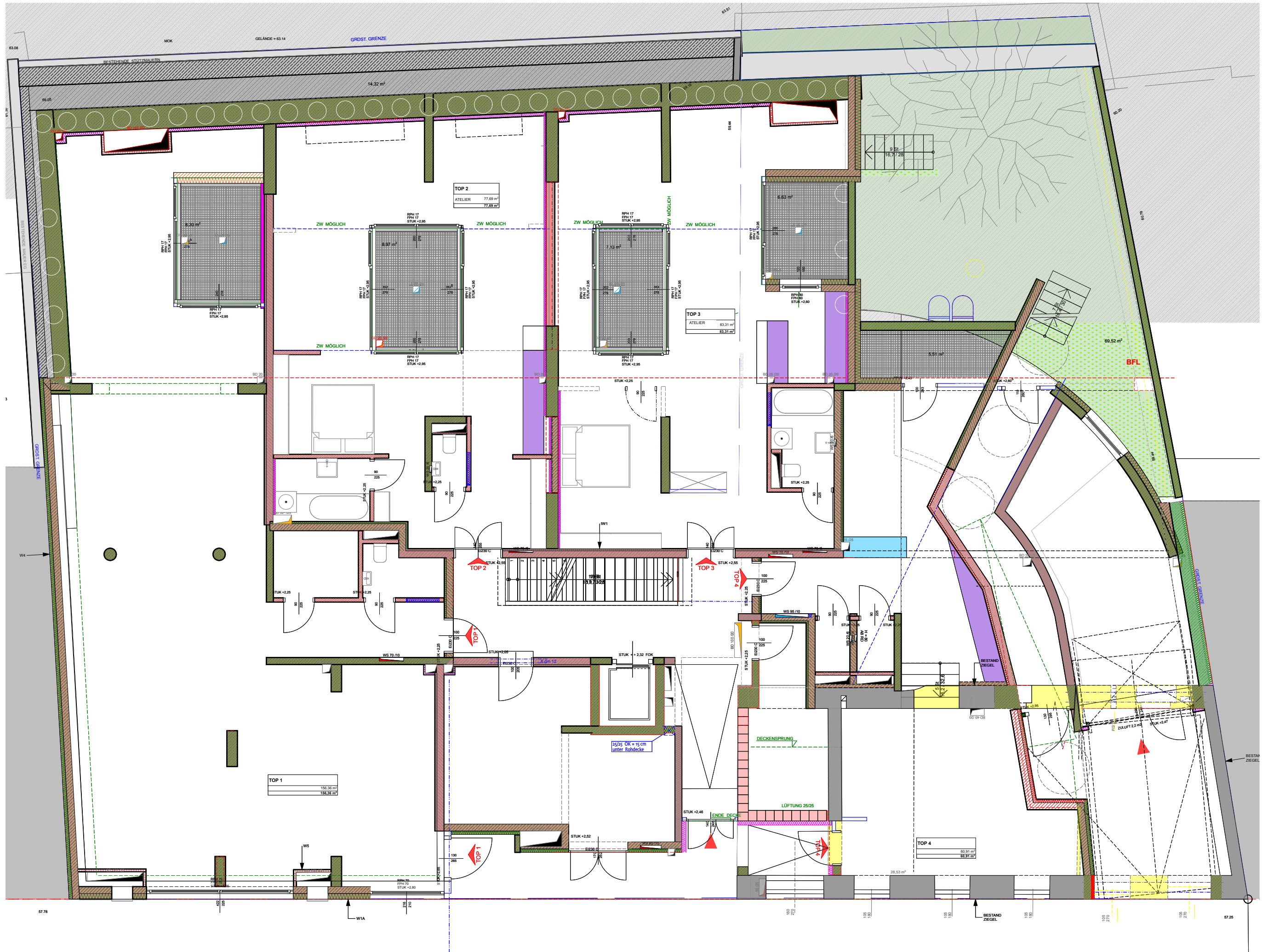
LINZERSTRASSE 306 GRUNDRISS EG
