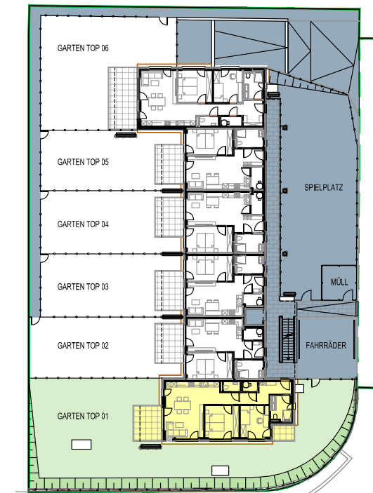
Übersicht Erdgeschoss
