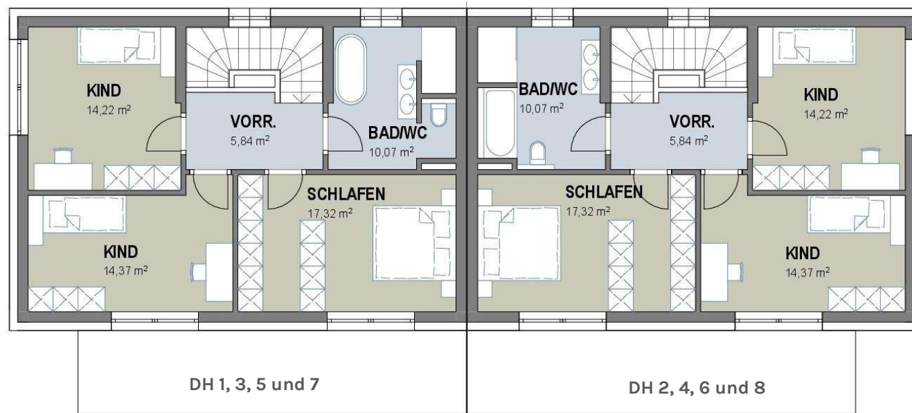
Obergeschoß Typ A und Typ B – ca. 60 m²
