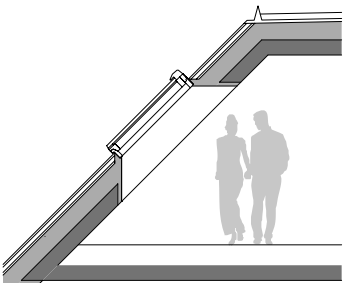
SCHNITT A
