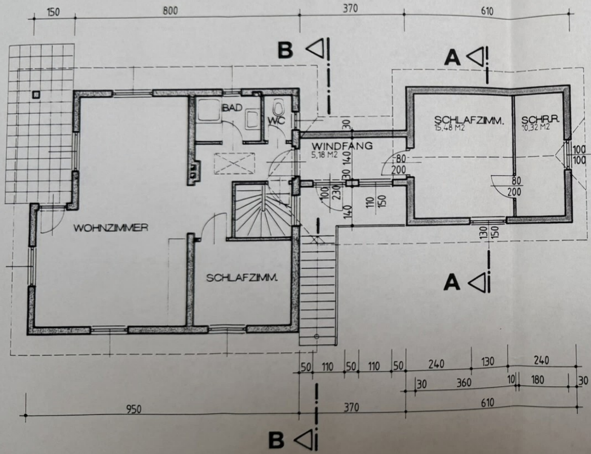
GRUNDRISS ERDGESCHOSS
