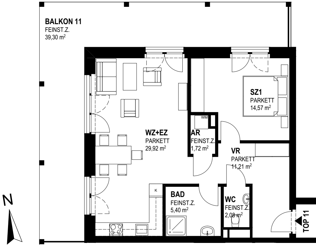
TOP 11 - 1.OG M1:100
