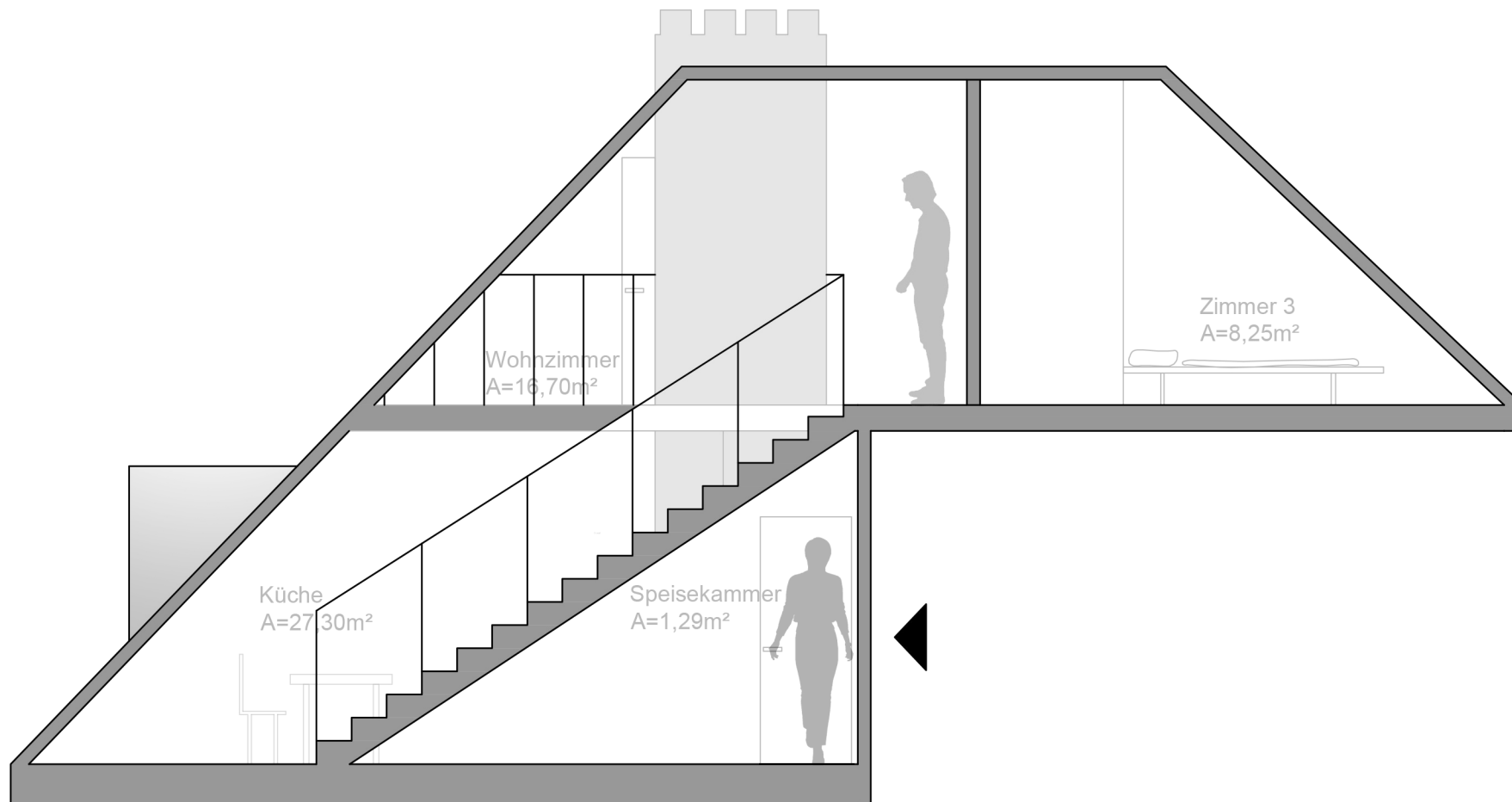
Schnitt AA
