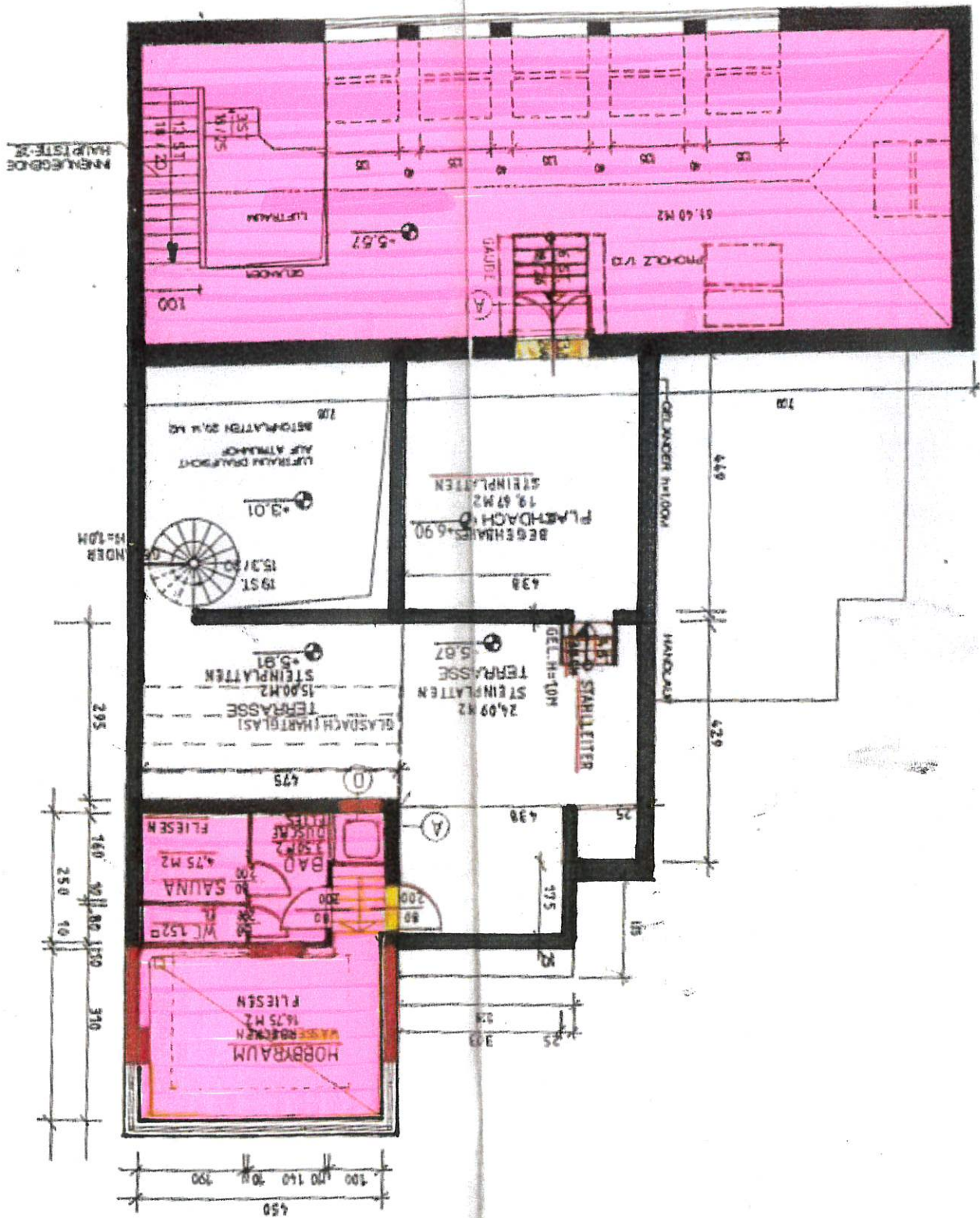
GRUNDRISS DACHGESCHOSS
