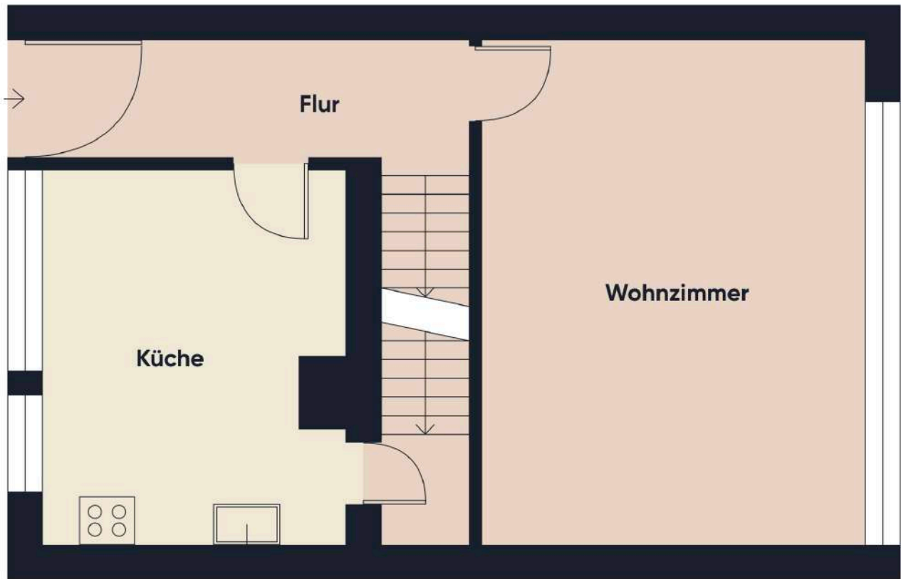
Grundrissplan ohne Maßstab EG
