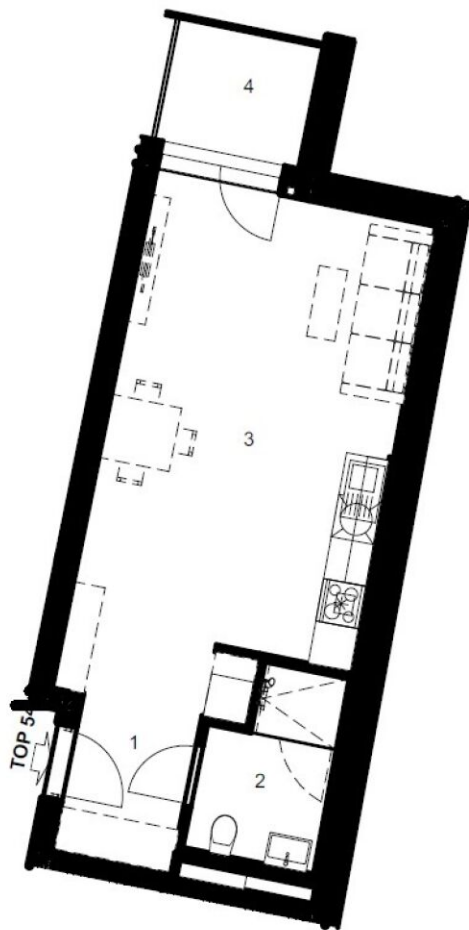
GRUNDRISS 4.OBERGESCHOSS
