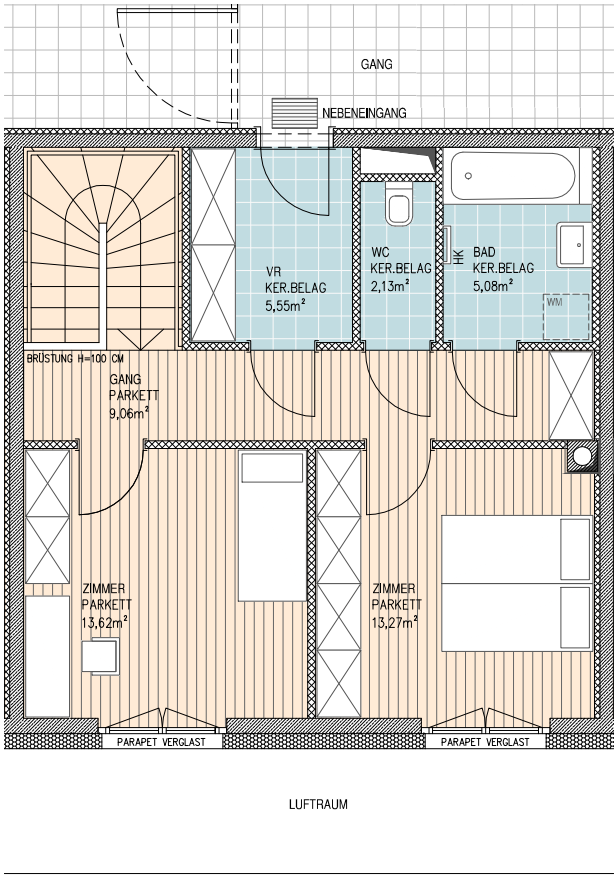
4.OG
