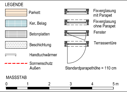
4.OG
