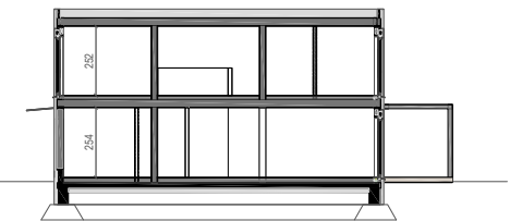
SCHEMATISCHER SCHNITT M 1:300
