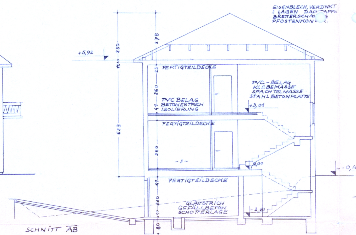
SCHNITT AB
