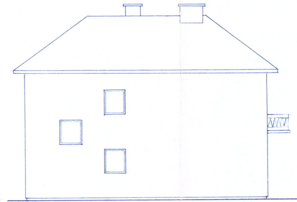
NW-ANSICHT
