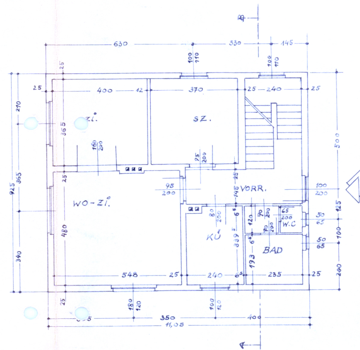
ERDGESCHOSS
