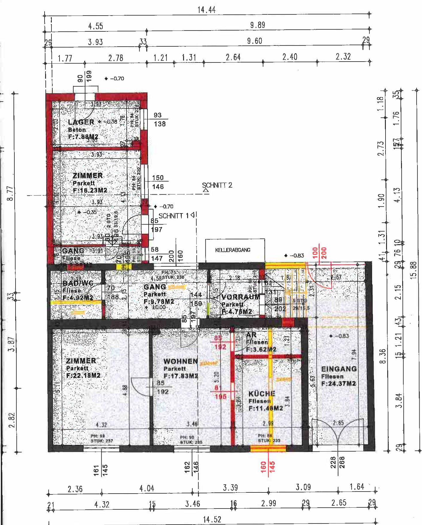
GRUNDRISS EG
