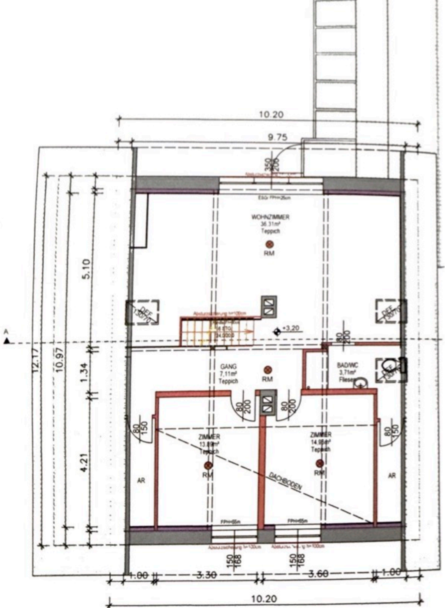
GRUNDRISS OBERGESCHOSS M1:100
