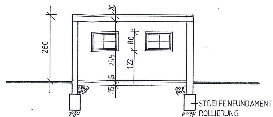
SCHNITT B-B M: 1/100
