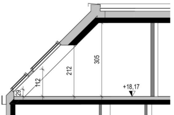
Schnitt 33.C
