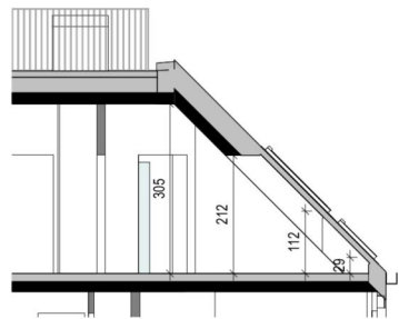
Schnitt 33.B
