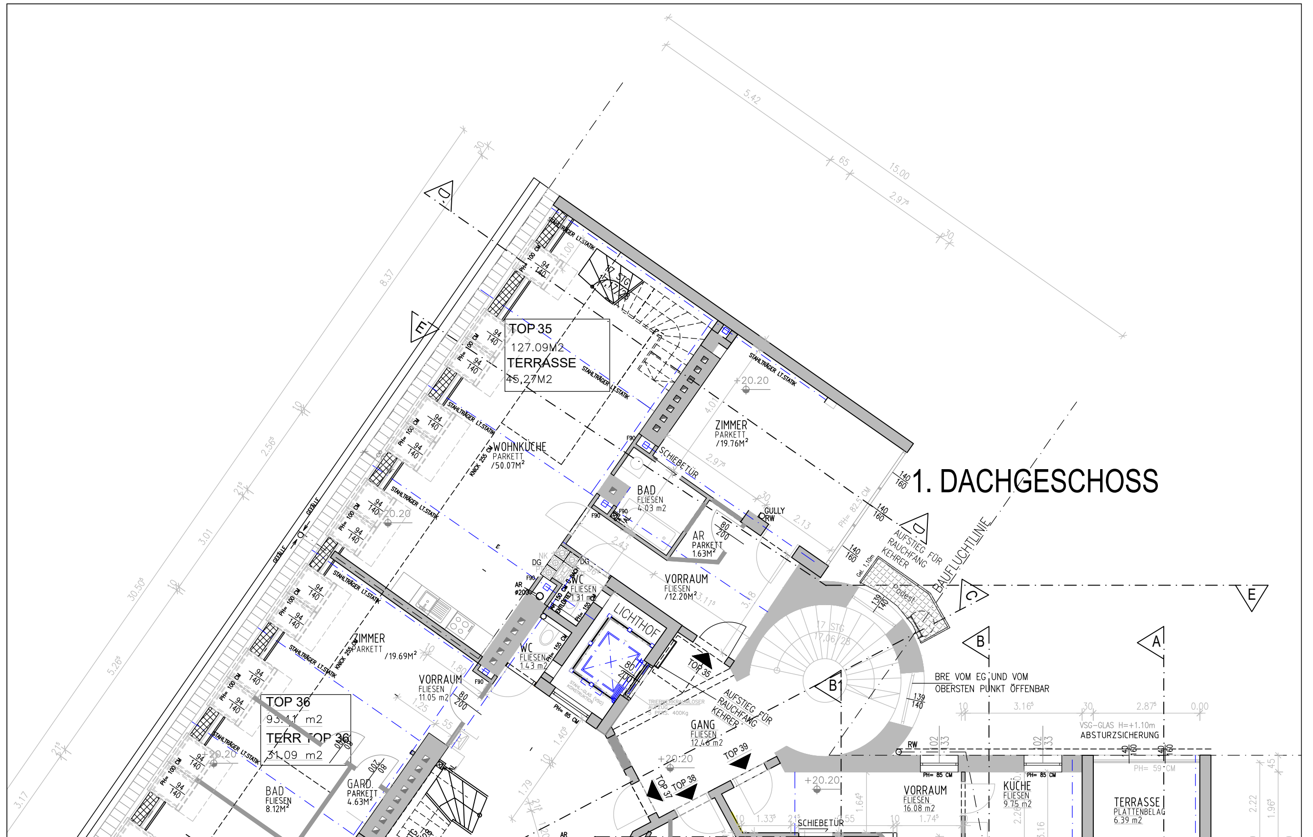
GRUNDRISS 1. DACHGESCHOSS
