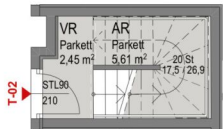
Grundriss EG:
