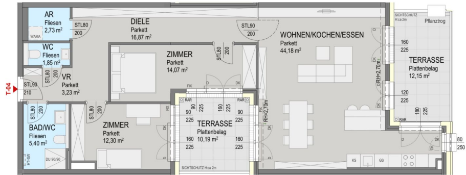
Grundriss 1 OG:
