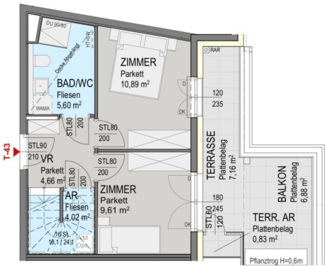
Grundriss 1 DG:
