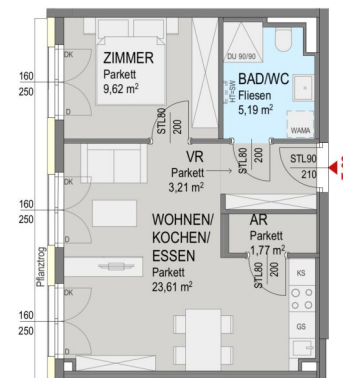
Grundriss 1 OG:
