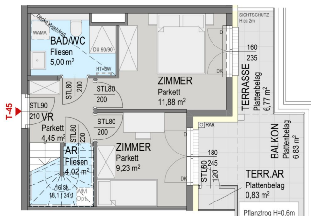
Grundriss 1 DG:
