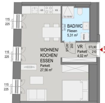
Grundriss 1 OG:
