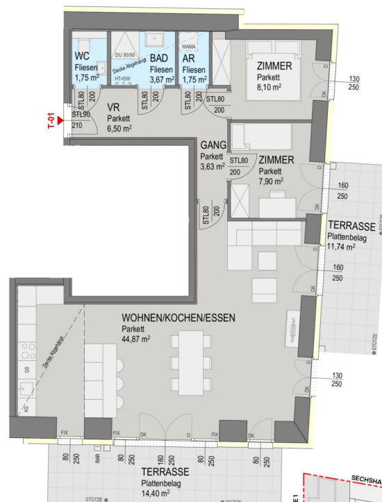
Grundriss EG:
