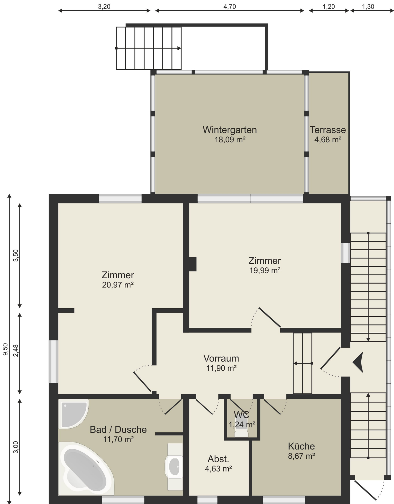
Erdgeschoss
