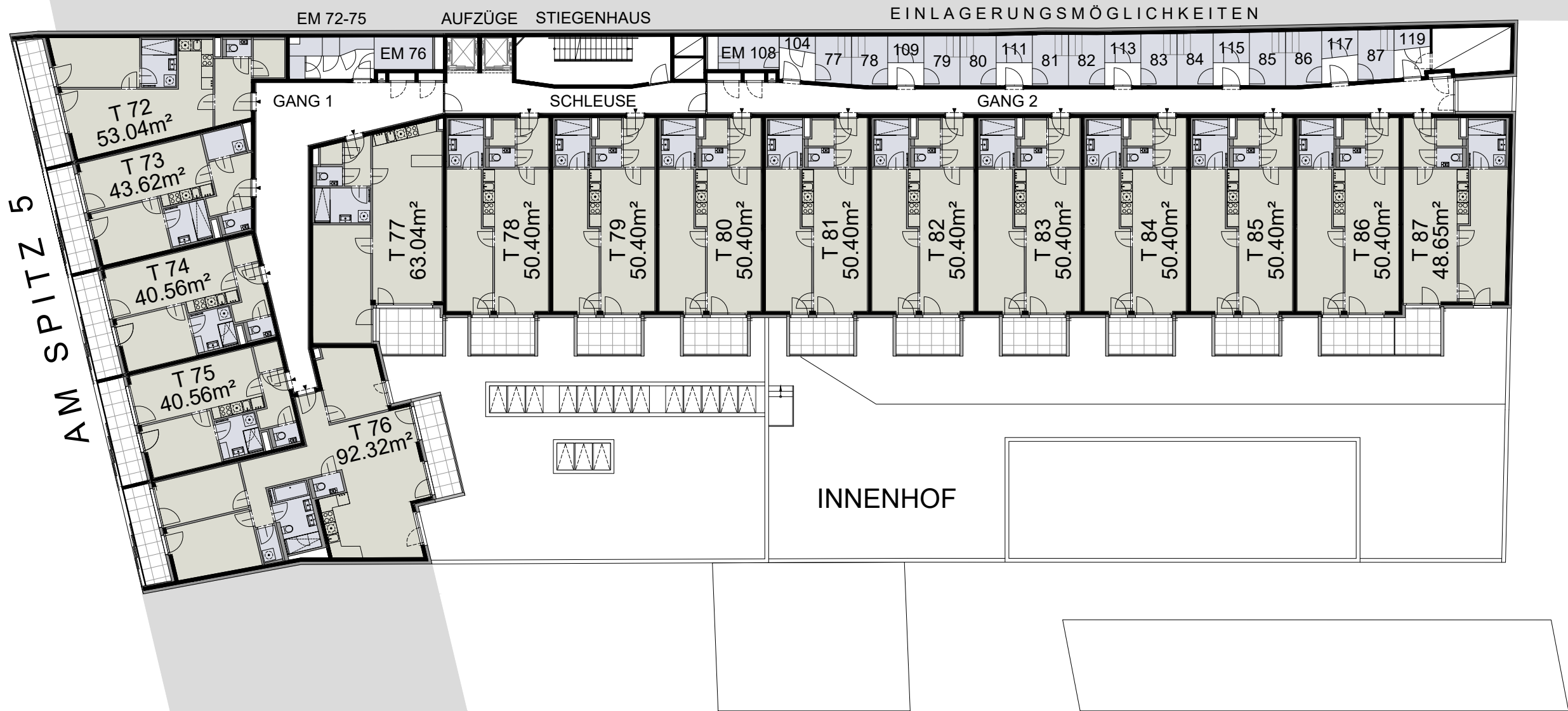
5. OBERGESCHOSS
