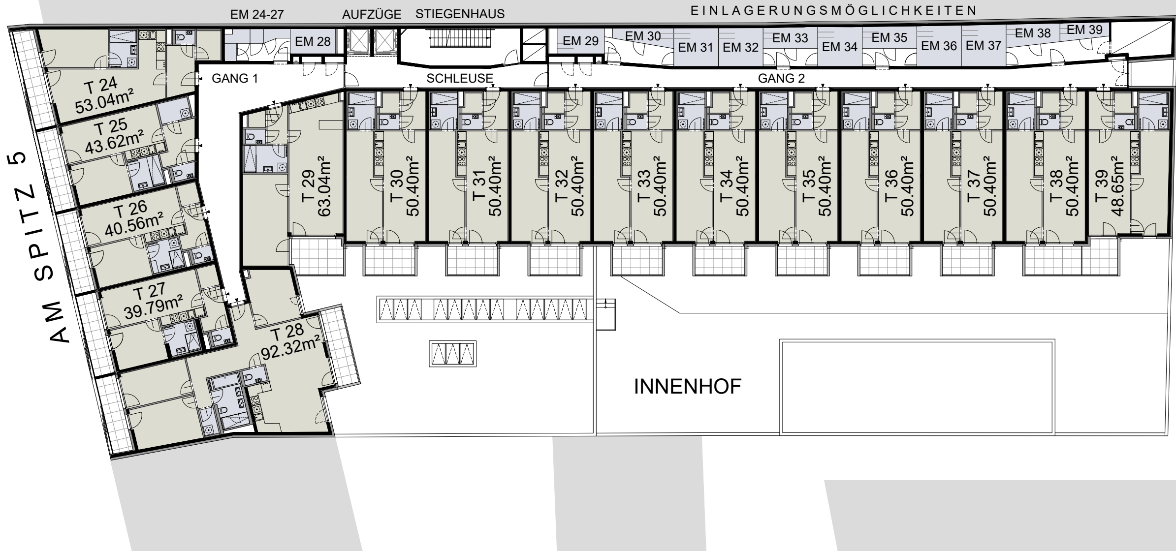
2. OBERGESCHOSS
