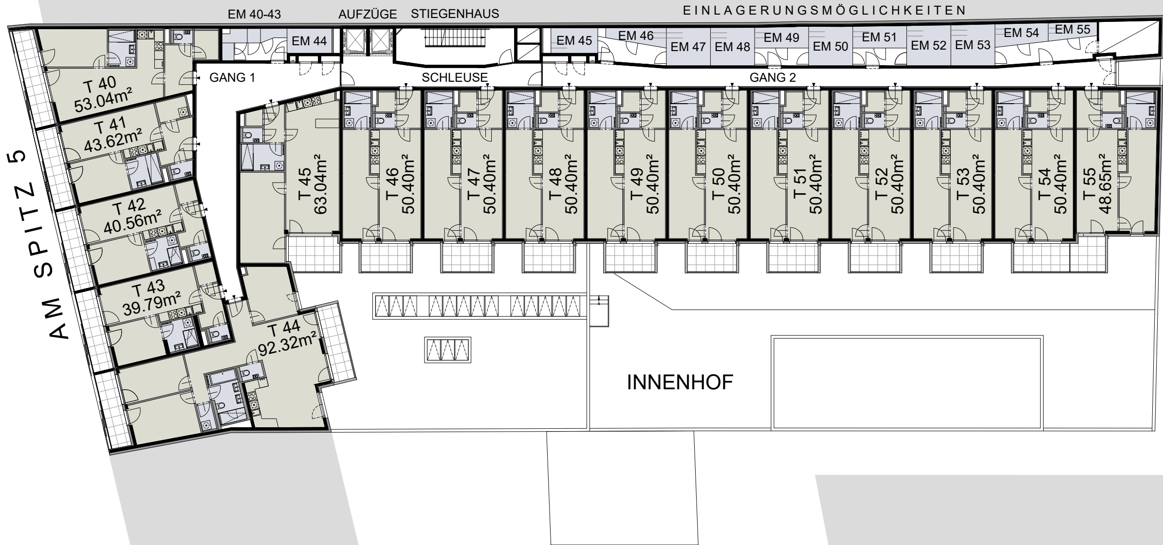
3. OBERGESCHOSS
