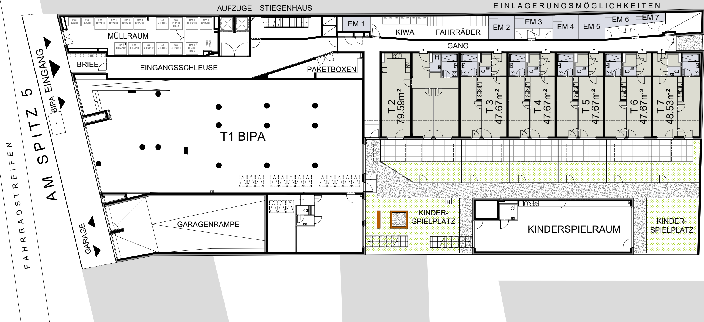
ERDGESCHOSS
