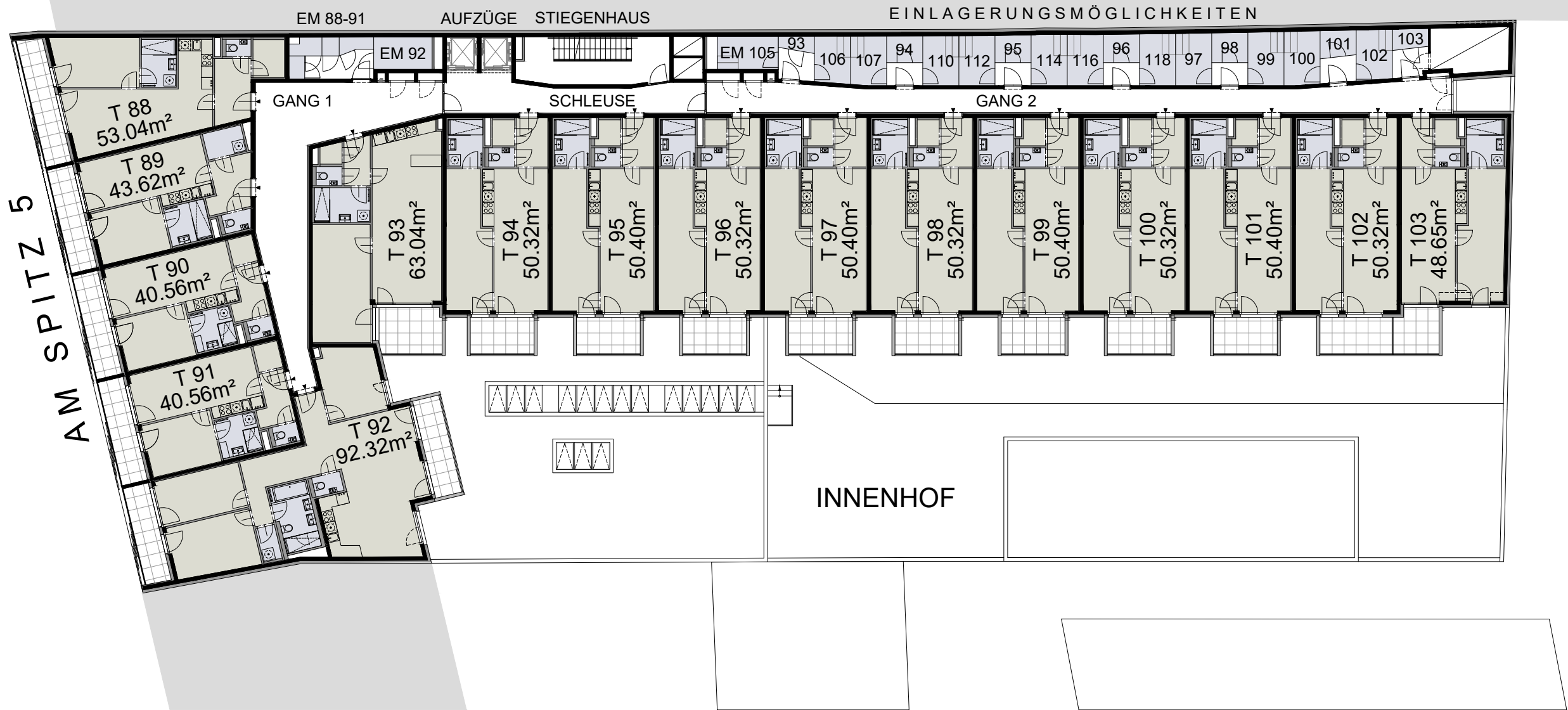
1. DACHGESCHOSS
