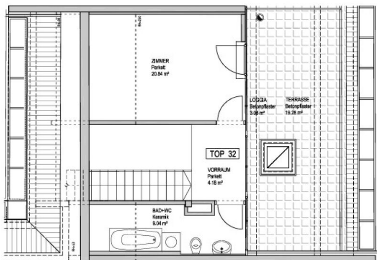
2. DACHGESCHOSS
