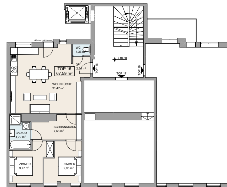
LAGEPLAN 1/200 PILGRAMGASSE 15
