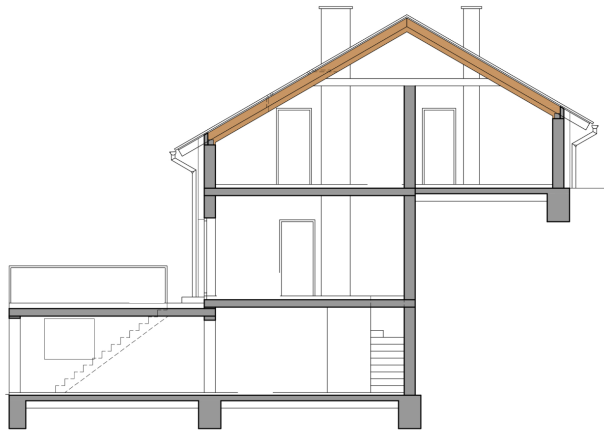
Schnitt
