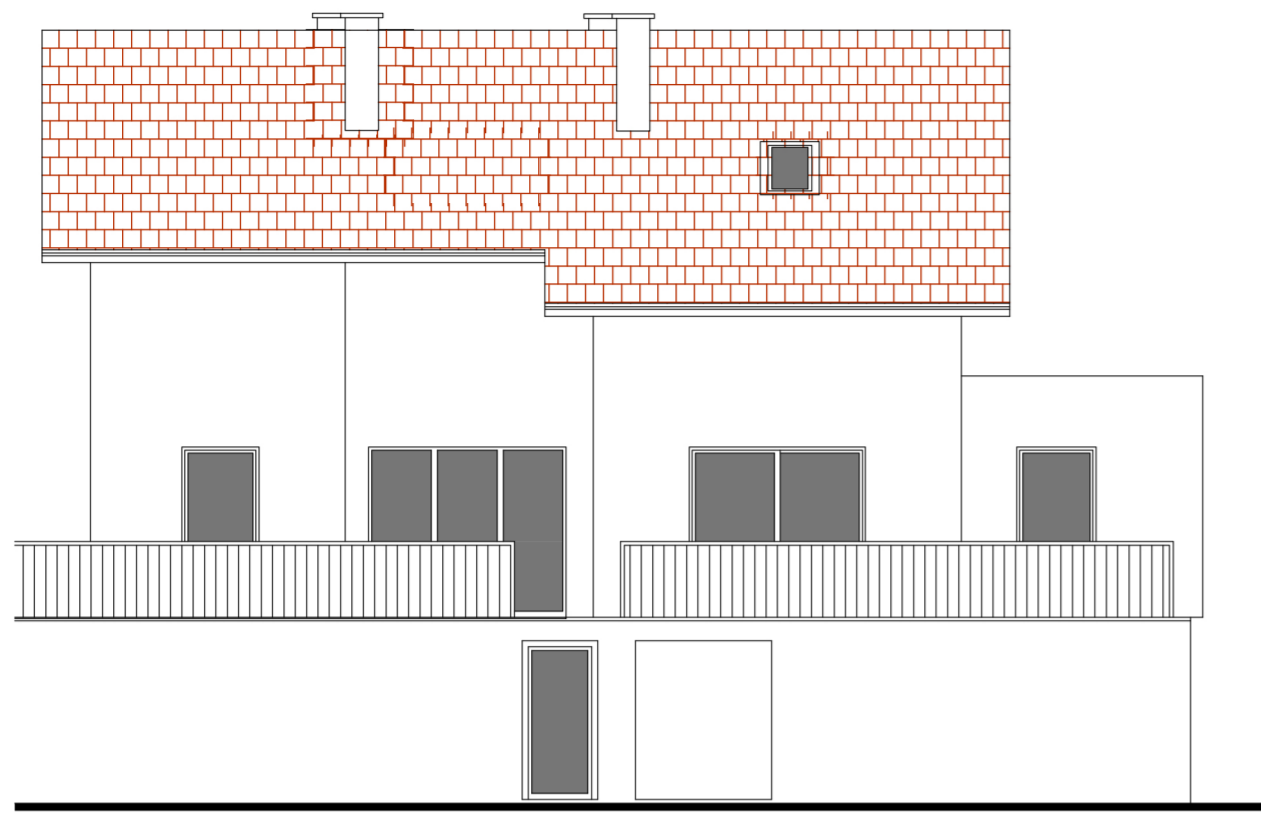
Südansicht
