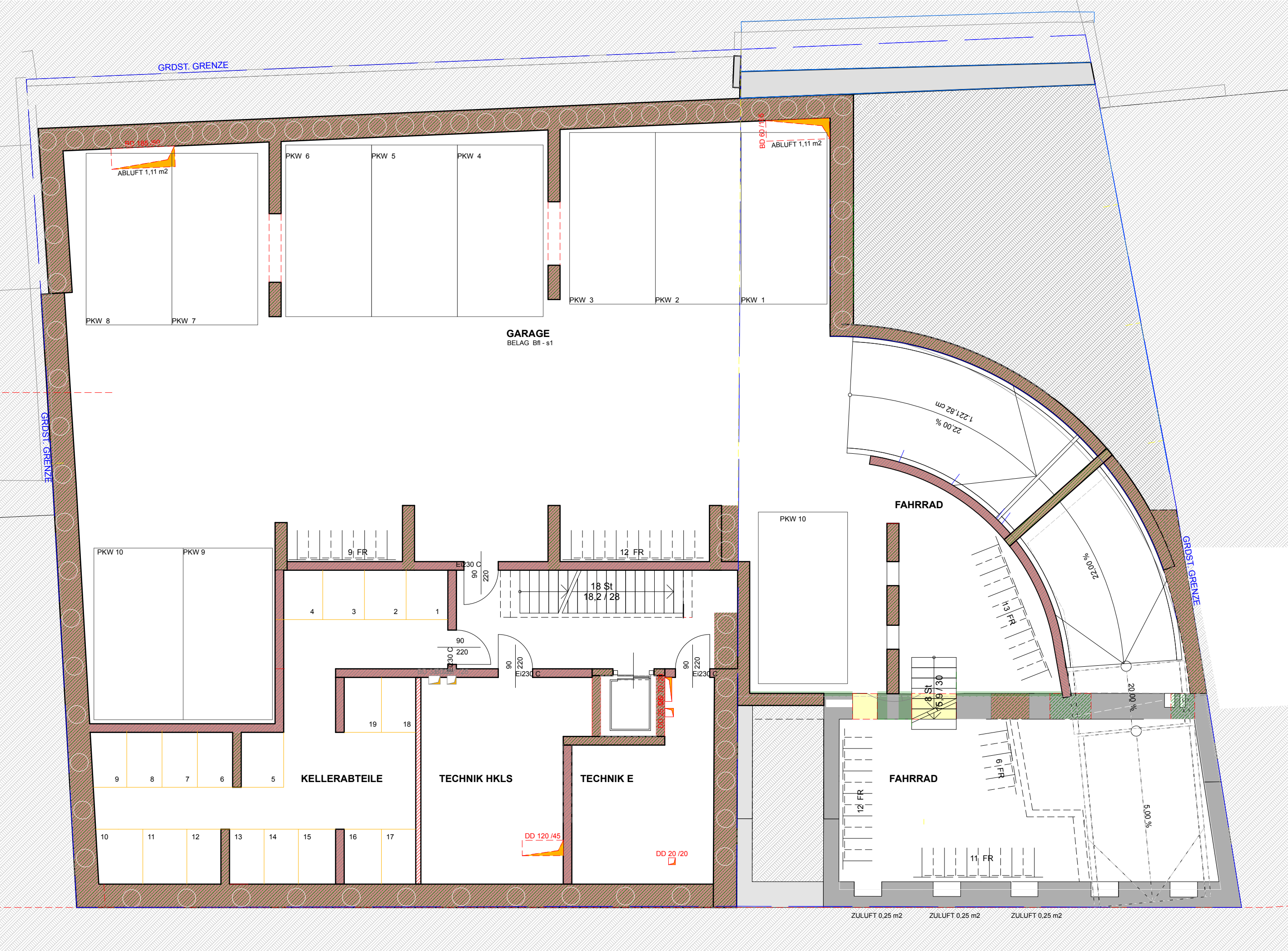
LINZERSTRASSE 306 GRUNDRISS EG
