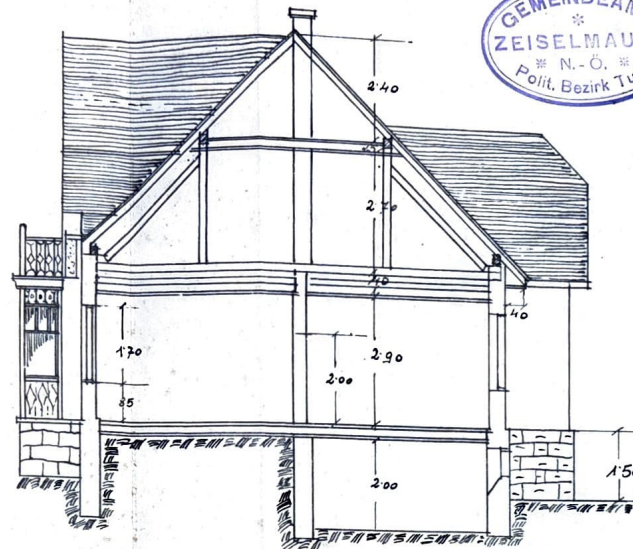
Schnitt.
