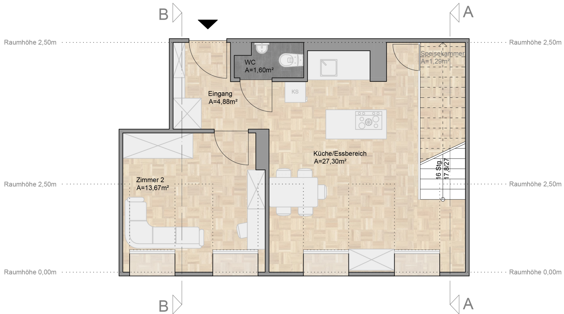
Grundriss: 1.DG
