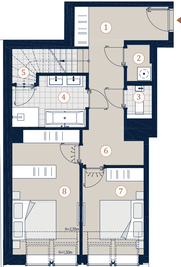
1.Dachgeschoß
