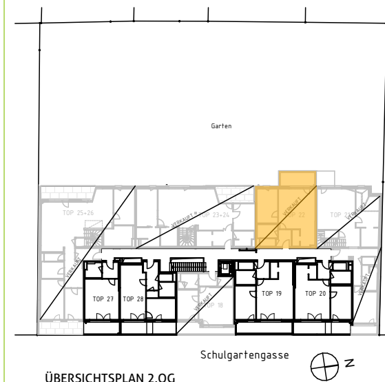
ÜBERSICHTSPLAN 2.OG
