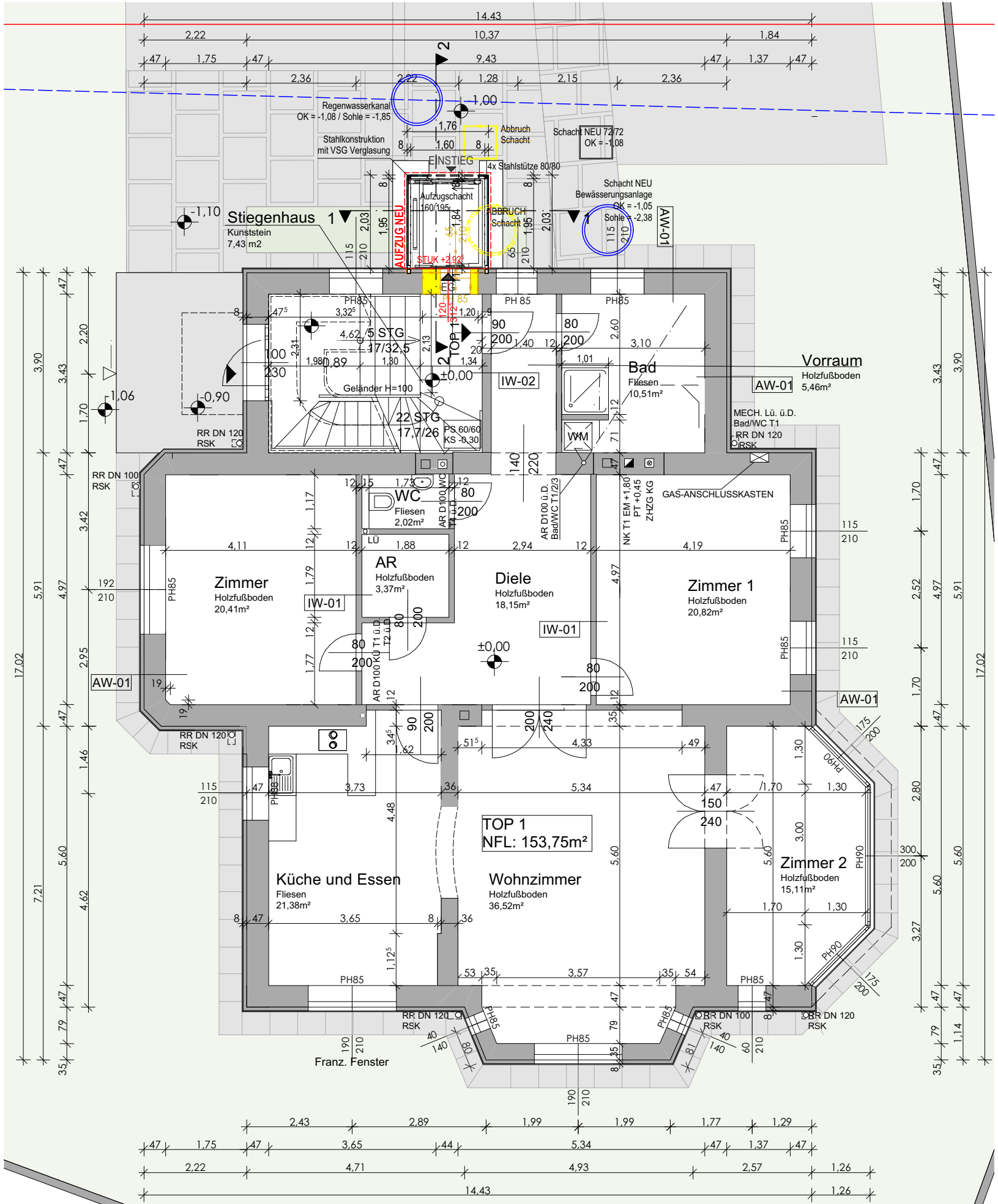
ERDGESCHOSS M 1:100
