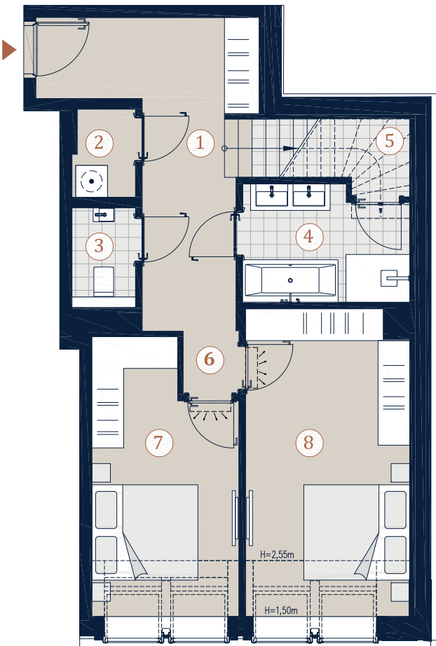
1.Dachgeschoß
