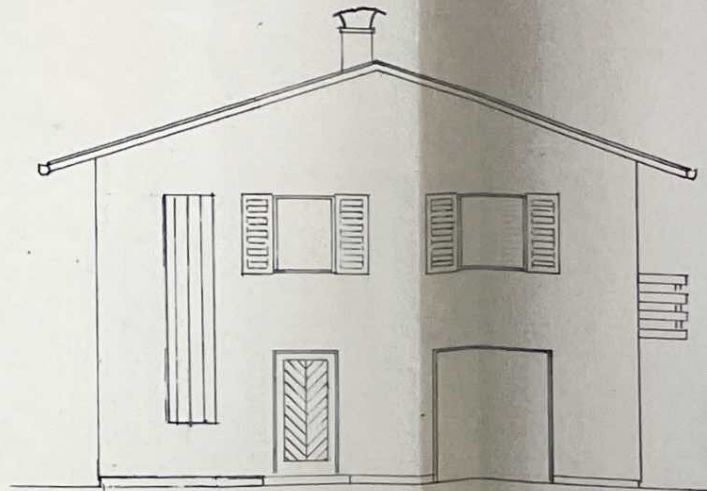
WESTANSICHT • 1:100
