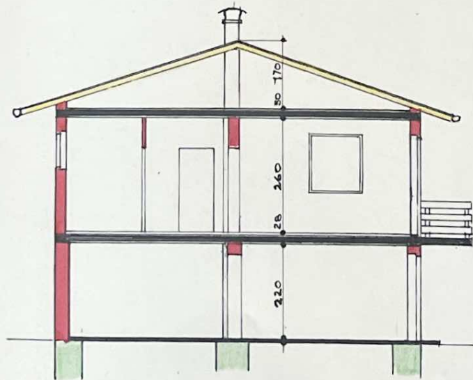
SCHNITT • 1:100
