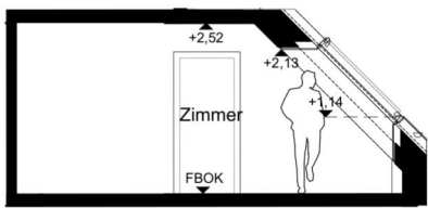
Schnitt
