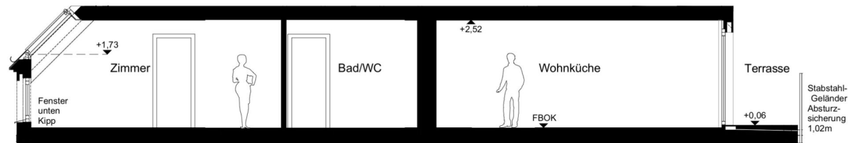
Schnitt
