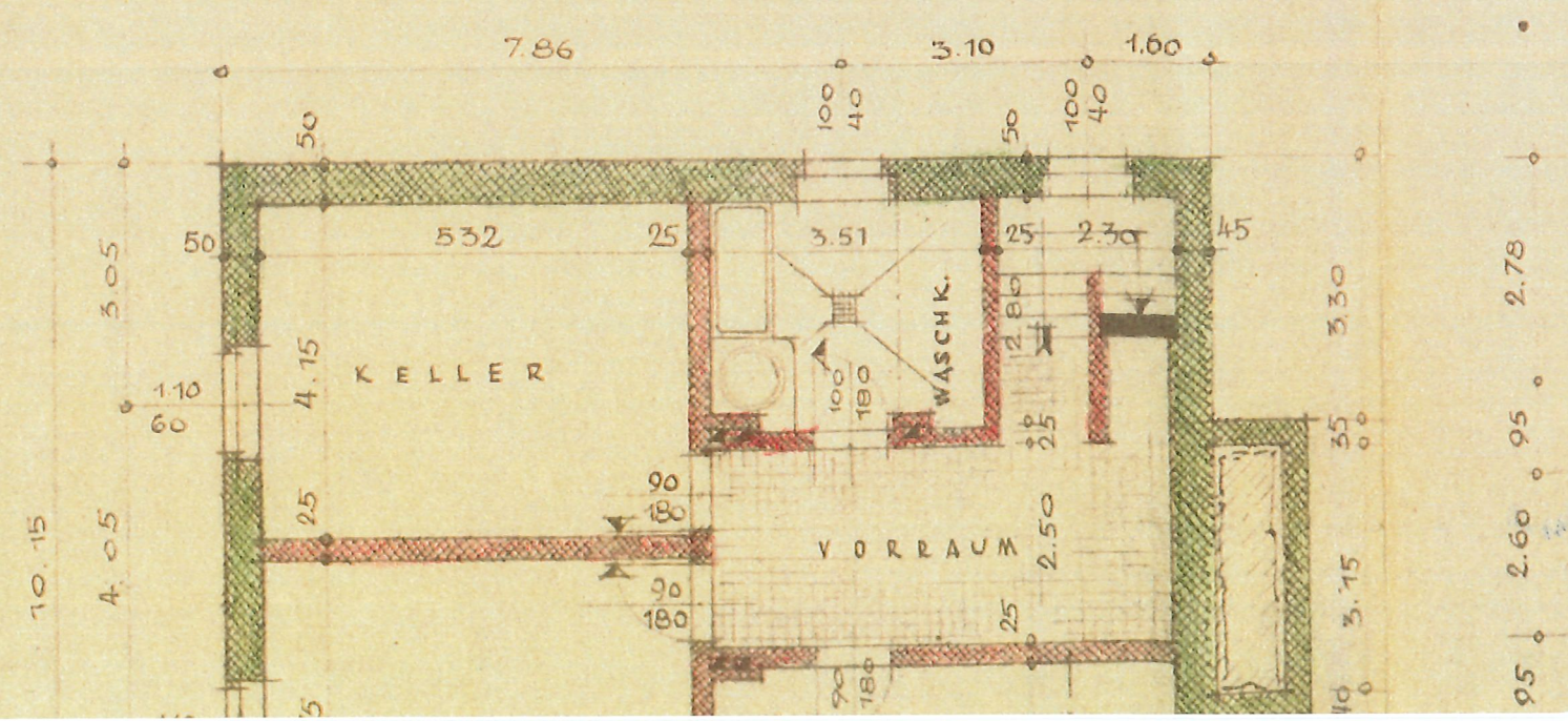
KELLERGESCHOSSGRUNDRISS.
