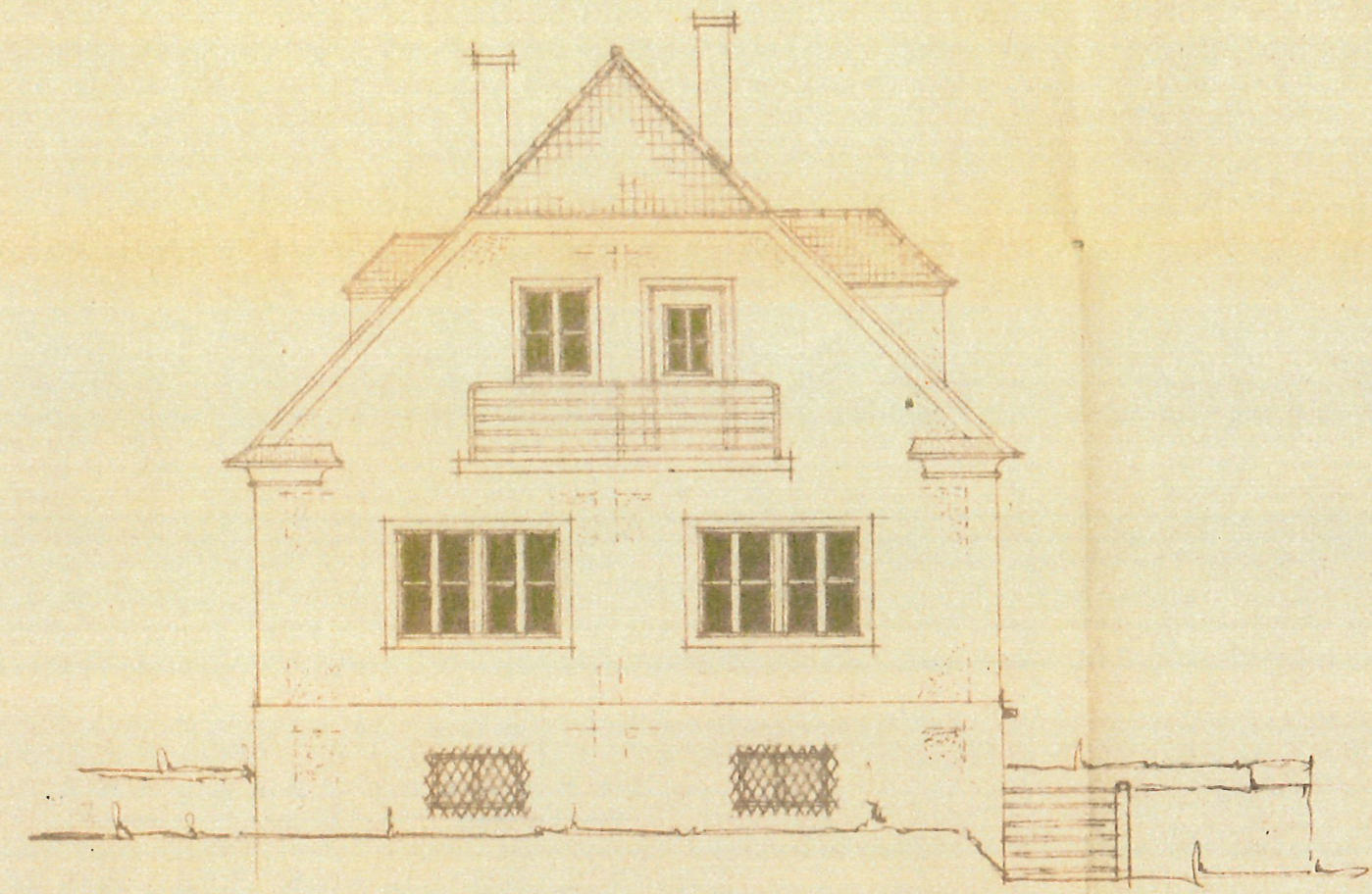
WESTANSICHT.
