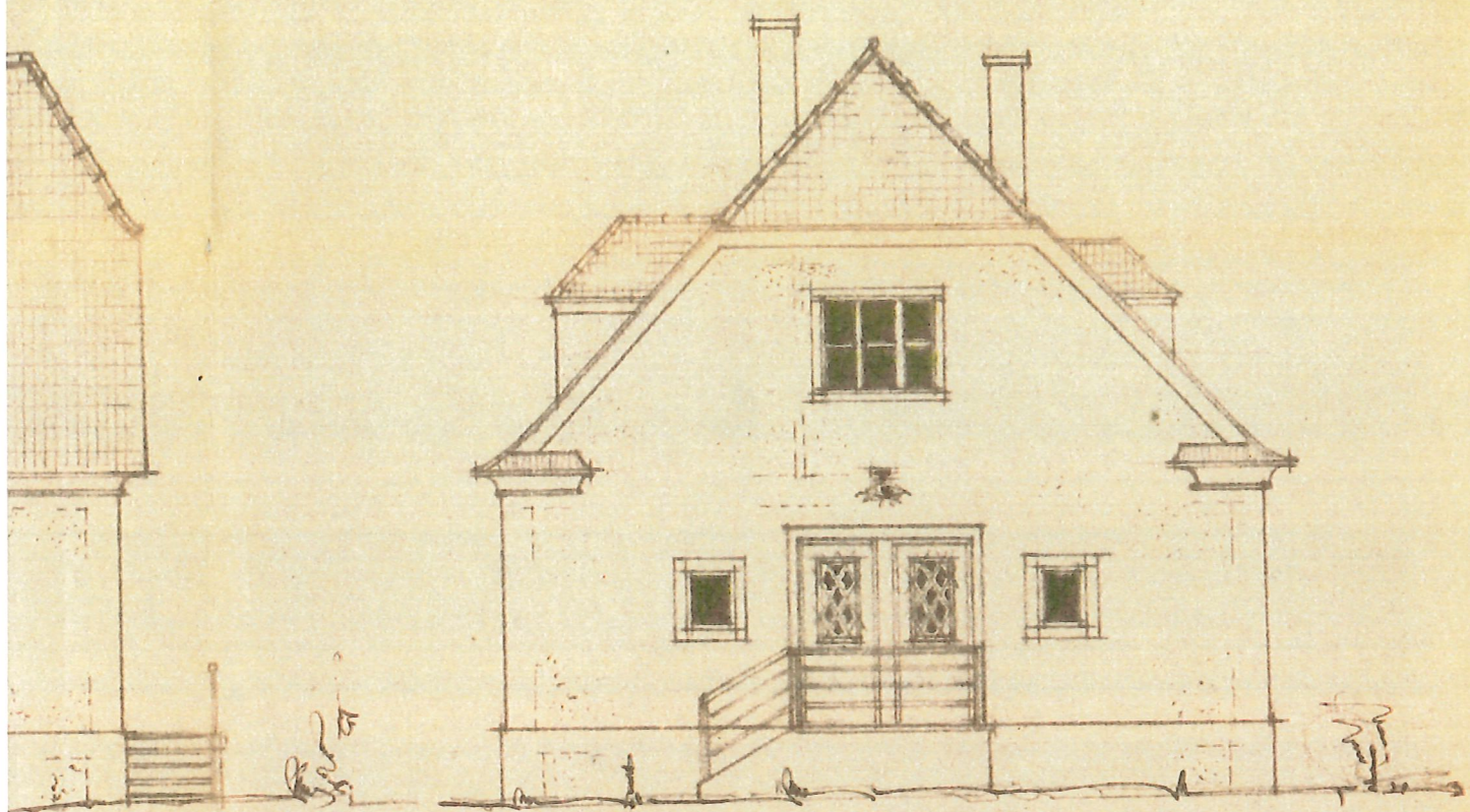
O STANSICHT
