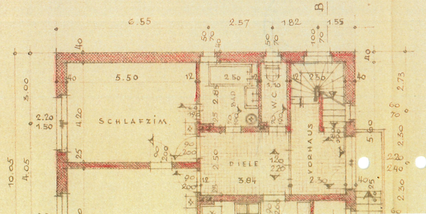
ERDGESCHOSSGRUNDRISS.
