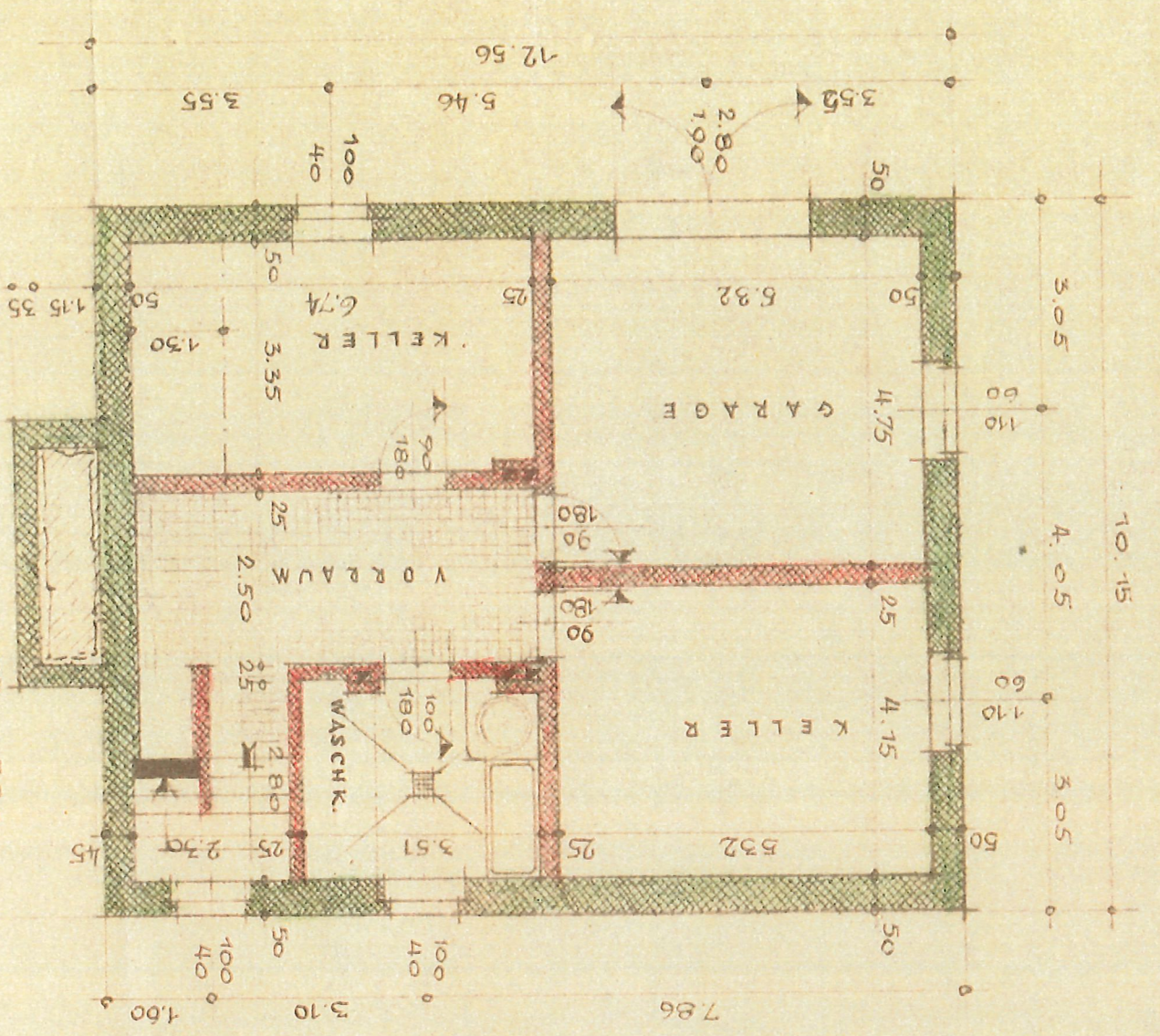
KELLERGESCHOSSGRUNDRISS.
