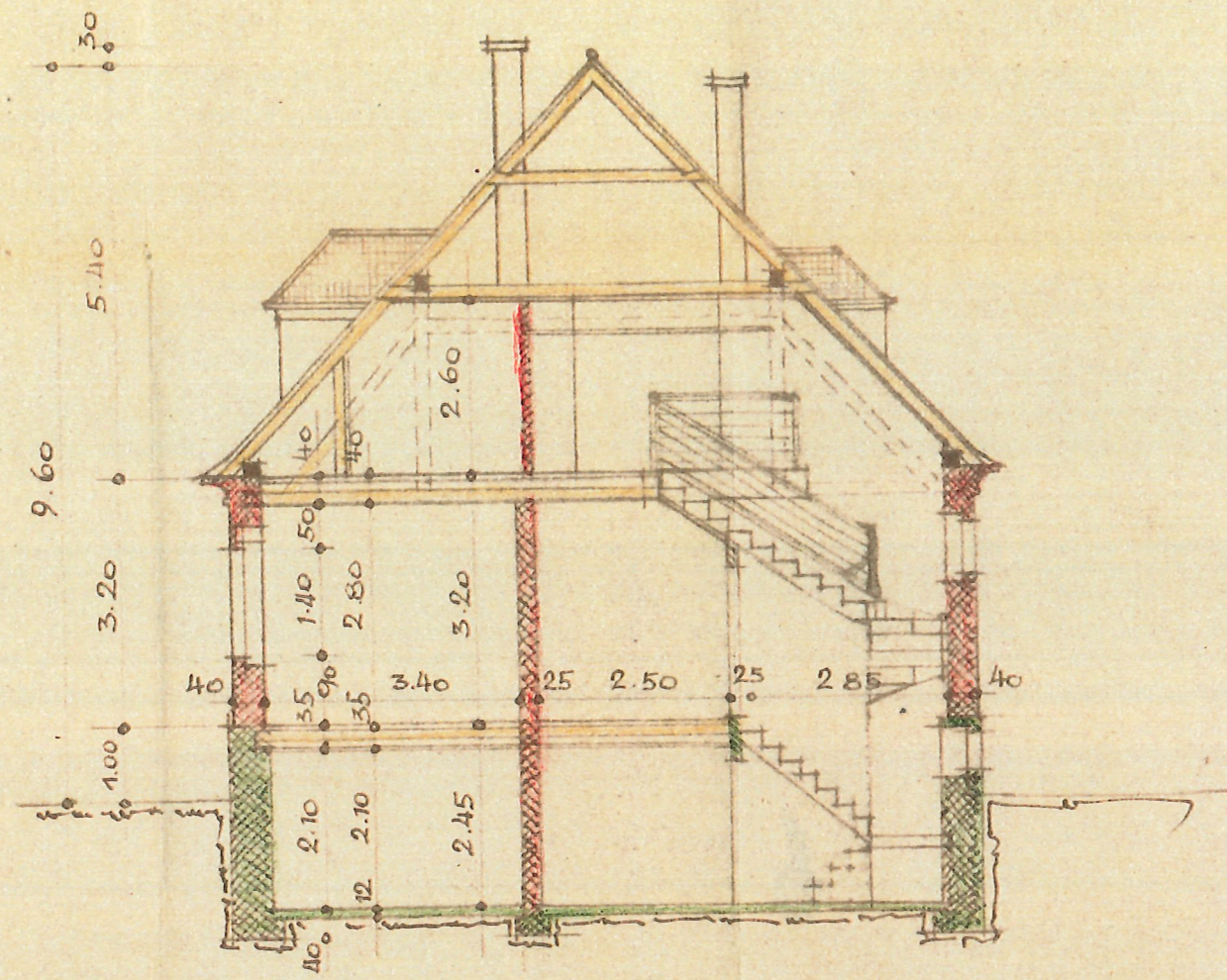
SCHNITT A-B
