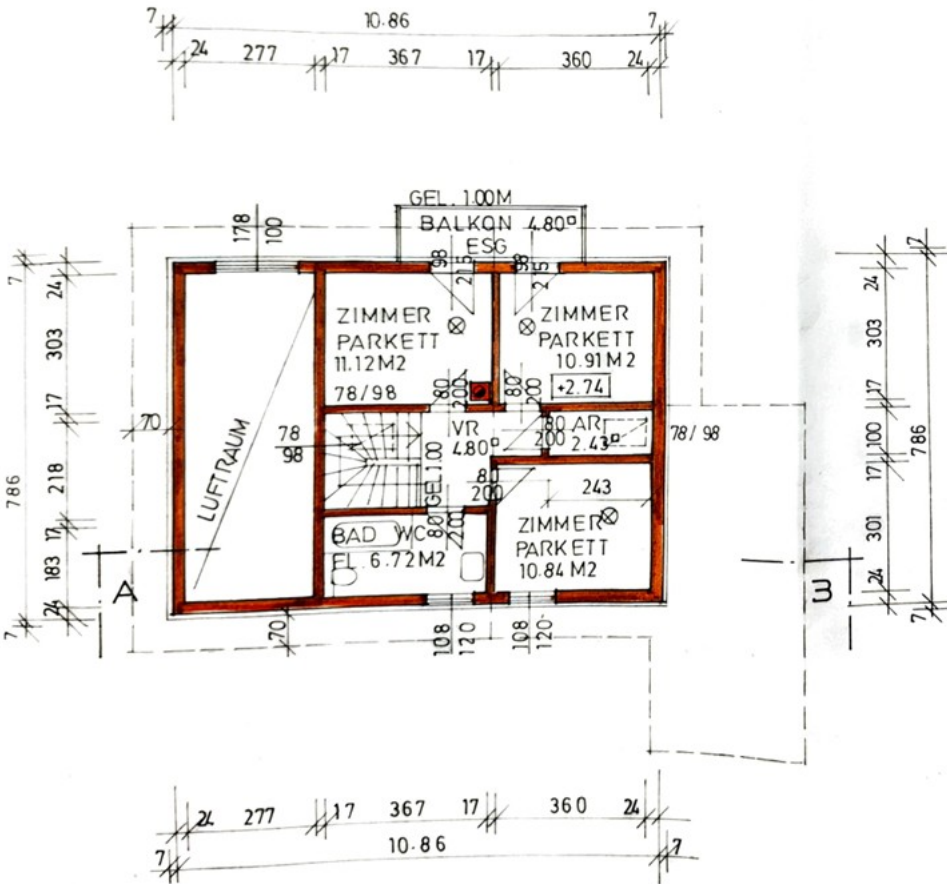
DACHGESCHOSS
