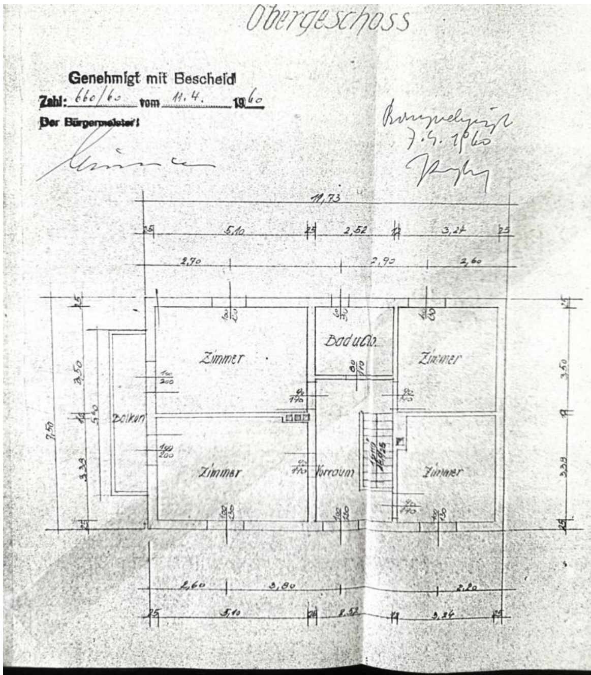
Obergeschoss
