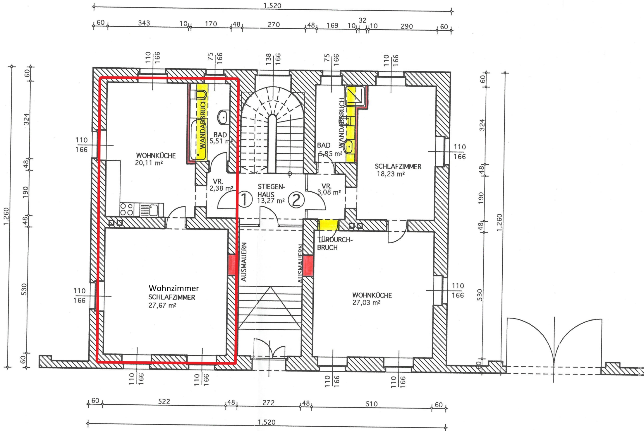
ERDGESCHOSS
