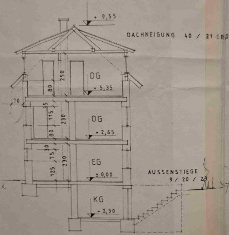
SCHNITT A - 3
