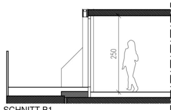
SCHNITT B1
