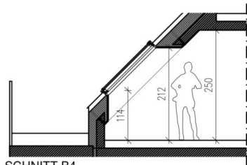
SCHNITT B4
