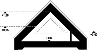
Schnitt 2
