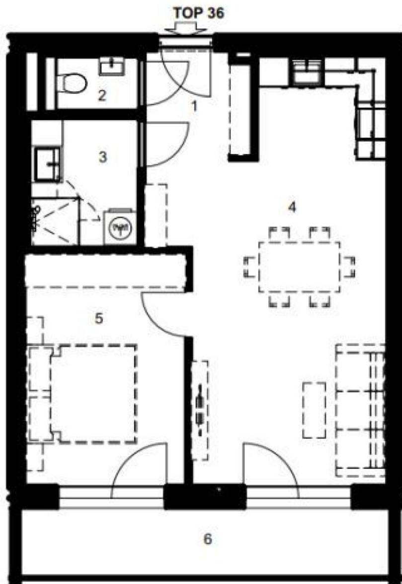
GRUNDRISS 3.OBERGESCHOSS
