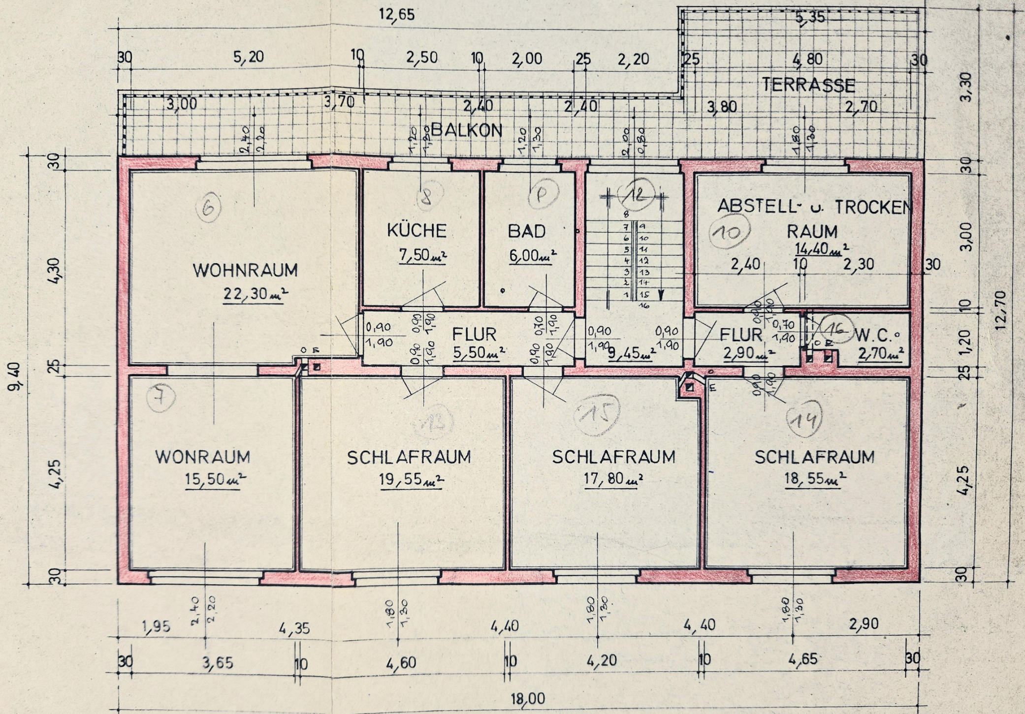
OBERGESCHOSSGRUNDRISS
