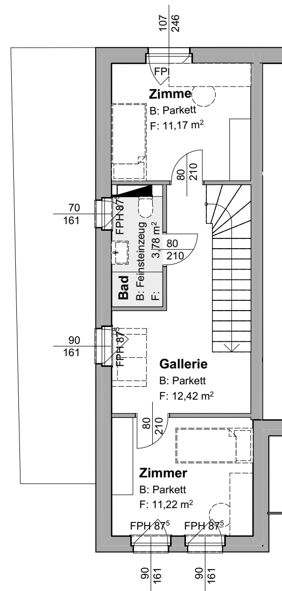
HAUS 5 2.OG M 1:100
