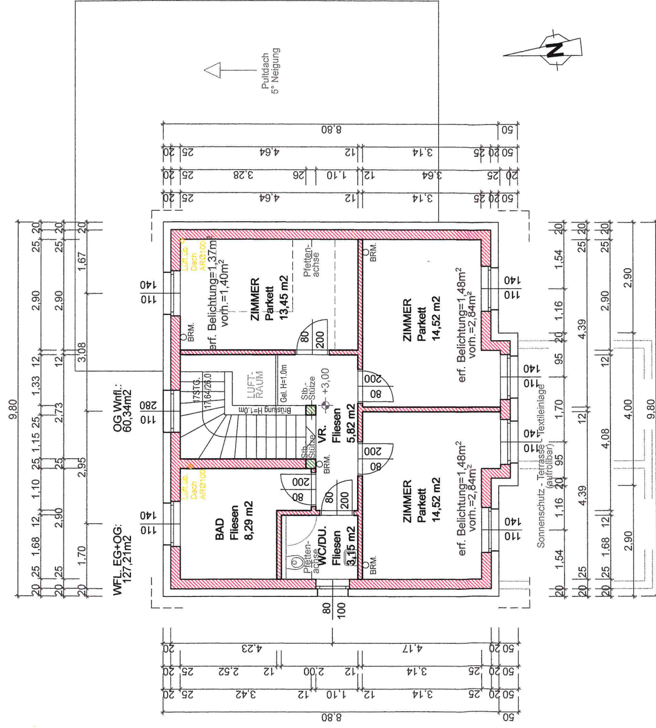
GRUNDRISS - OBERGESCHOSS 1 : 100
